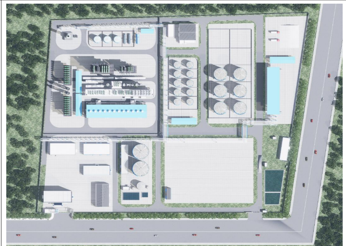
6 万吨生物质新能源项目-总平面布置图
