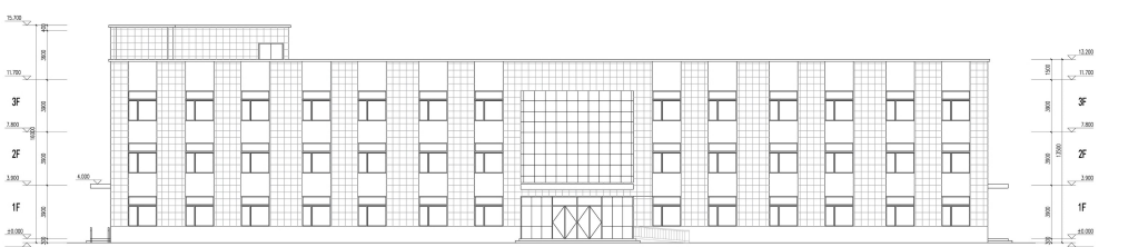
南立面图
