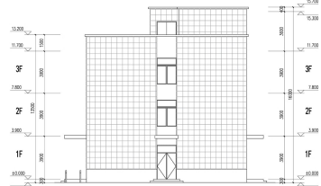
东立面图
