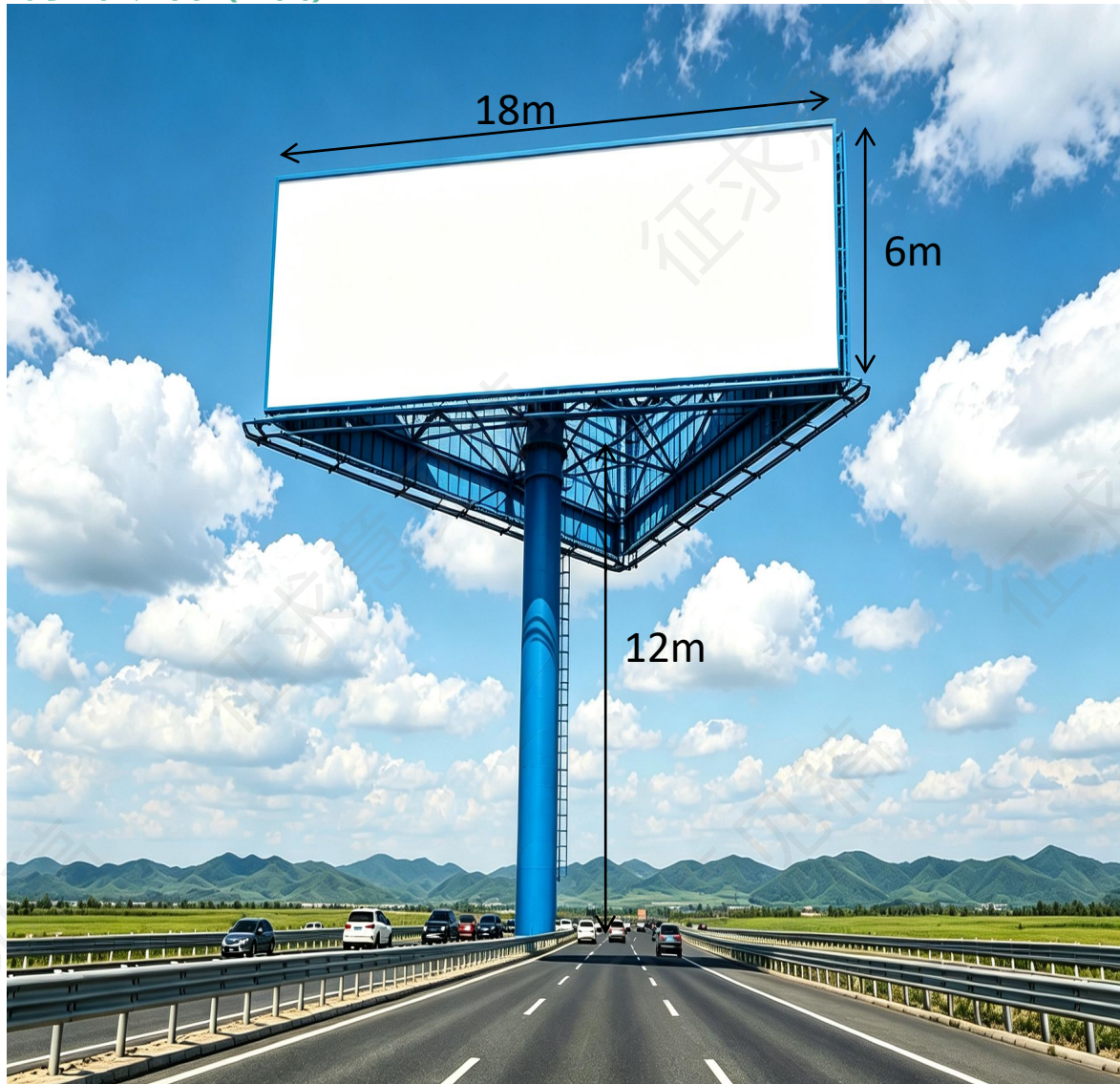
规划高立柱广告尺寸示意图二
